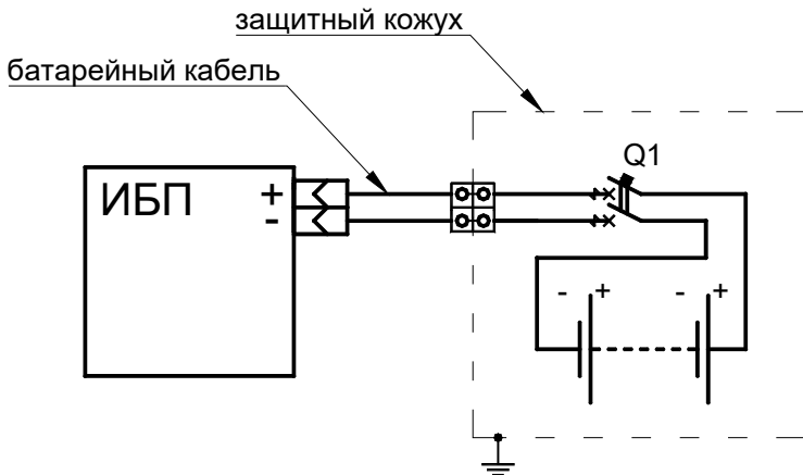
Рисунок 11 – Схема электрическая подключения аккумуляторной батареи к ИБП
