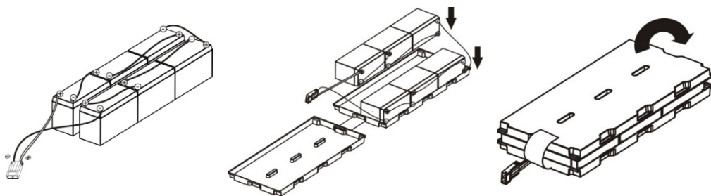
Рисунок 21 – Последовательность установки аккумуляторов в контейнер ИБПАТС 3000 R-BE
